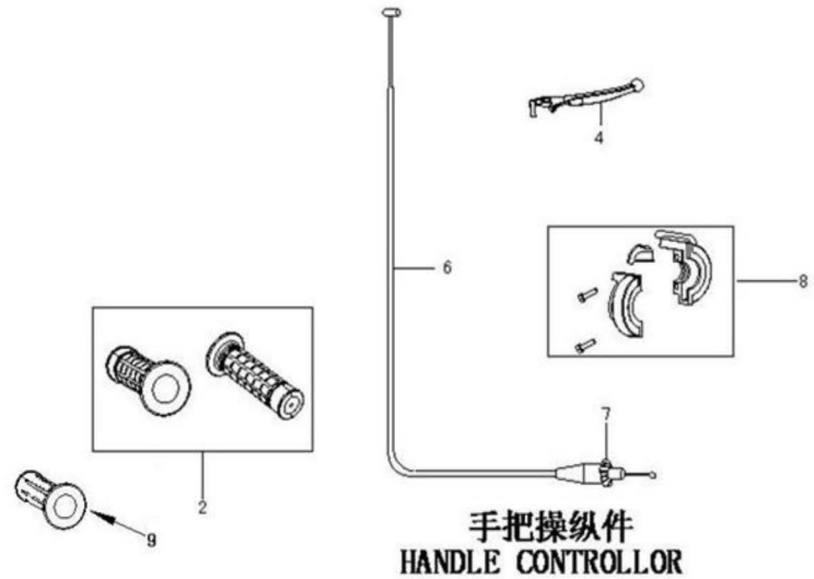
手把操纵件 HANDLE CONTROLLER
