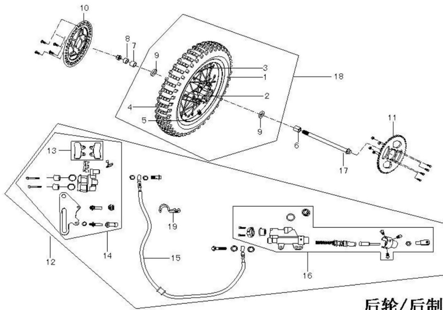
后轮/后制动器 RR. WHEEL/RR. BRAKE ASSY
