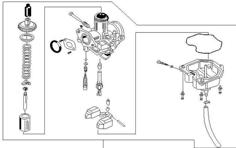
化油器 CARBURETOR
