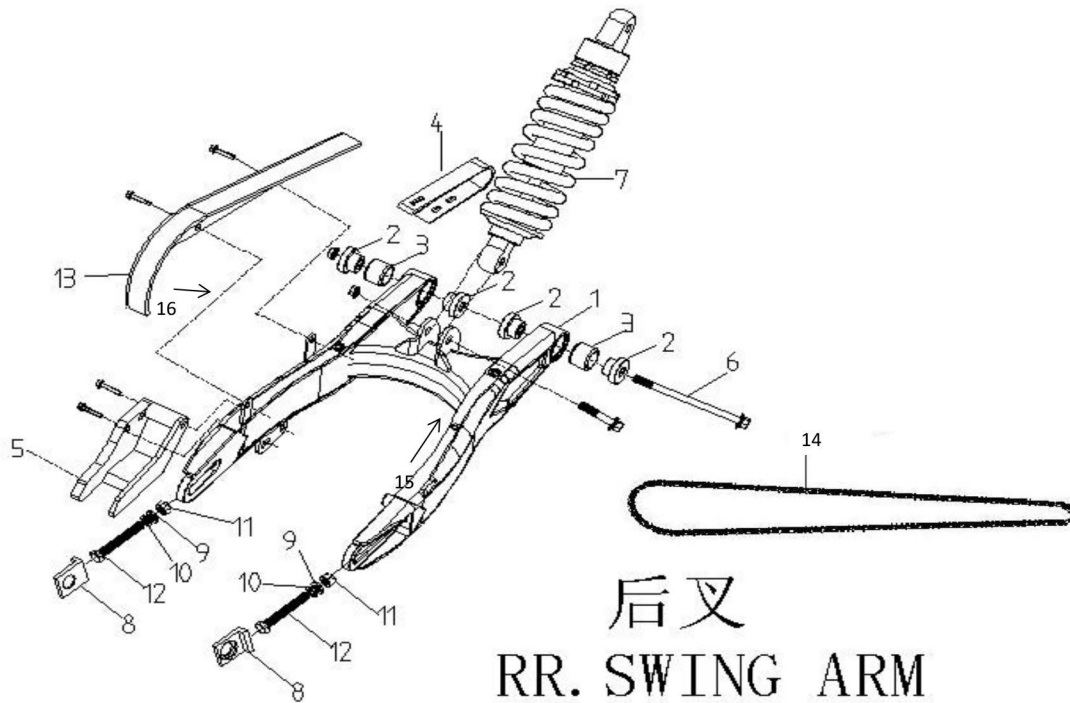
后叉 RR. SWINGARM
