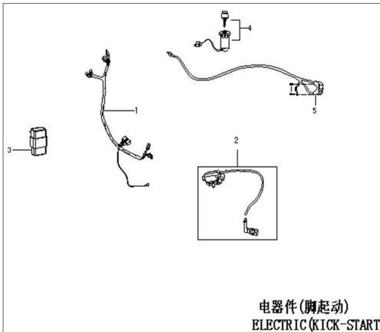
电器件 ELECTRIC
