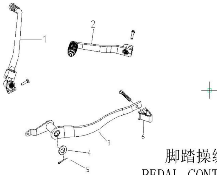
脚踏操纵件 PEDAL CONTROLLER
